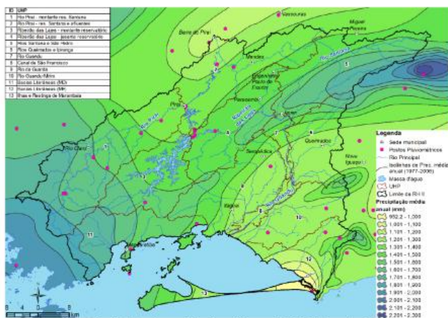
Figura 5 – Isoietas de precipitação média anual (PERH Guandu, 2018).
