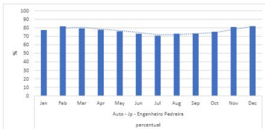
Figura 11 – Umidade relativa do ar na estação Auto JP Engenheiro Pedreira (INEA, 2020).
