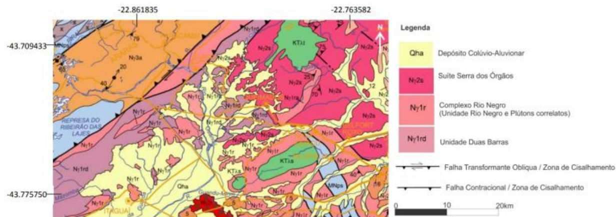
Figura 13 – Geologia Regional do Município de Queimados (CPRM, 2001).
