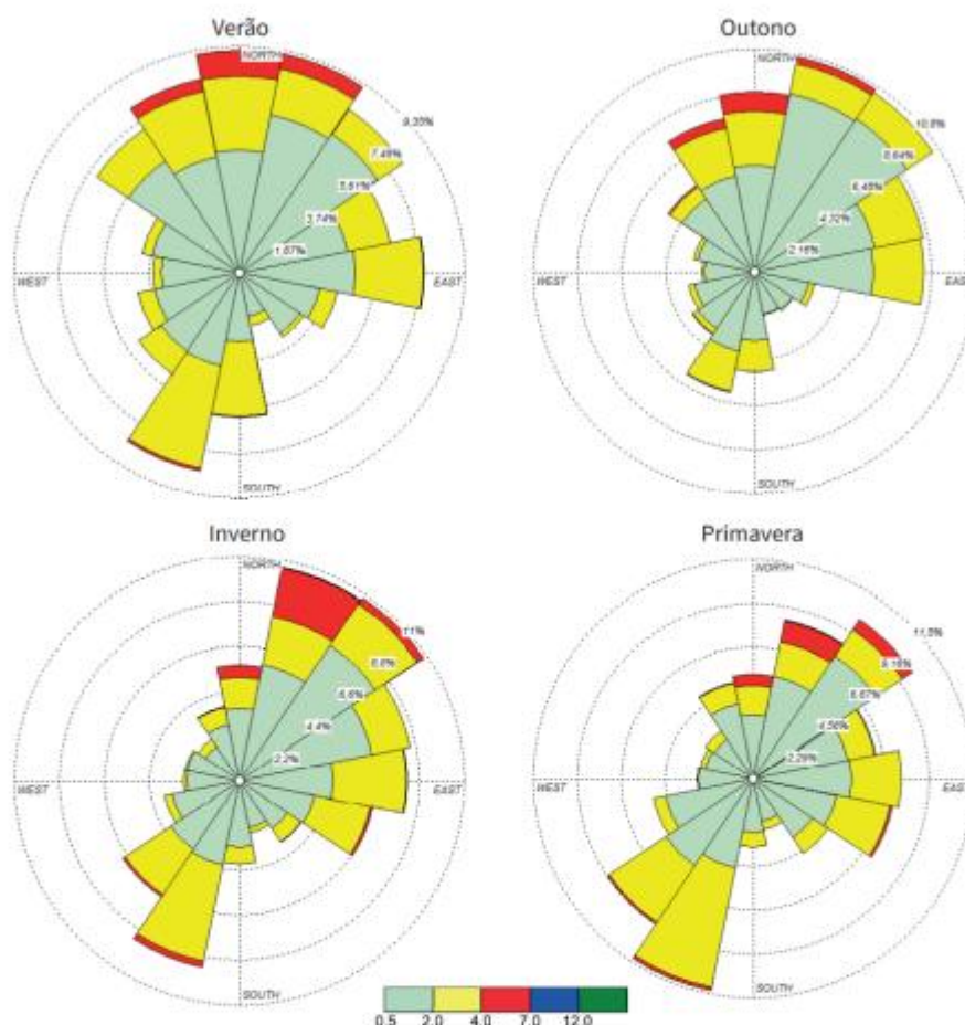
Figura 9 - Direção e intensidade do vento na estação Engenheiro Pedreira (INEA, 2020).
