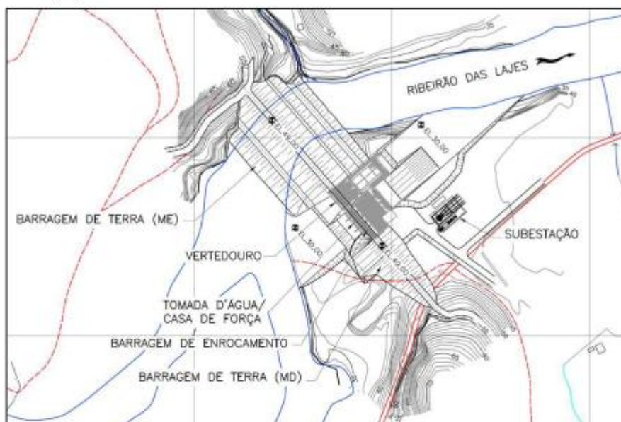
Figura 28 – Arranjo geral do barramento (Paracambi Energética, 2024).
