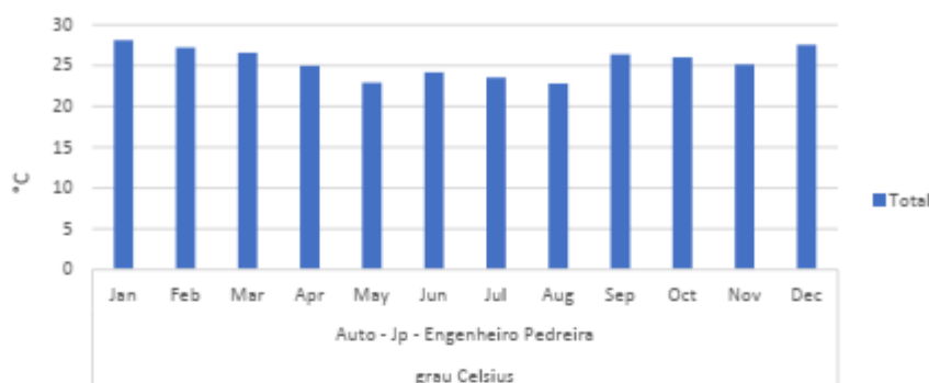
Figura 8 – Temperatura média registrada na estação Auto – Jp – Engenheiro Pedreira no ano de 2020 (INEA, 2020).
