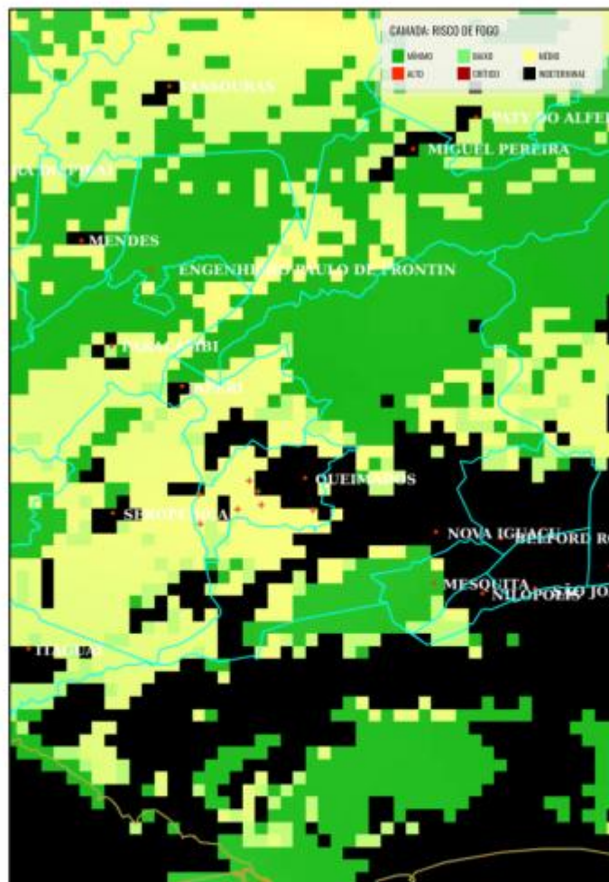
Figura 32 – Áreas de risco de fogo no município de Queimados considerando o ano de 2024 (INPE, 2025) 1 .
