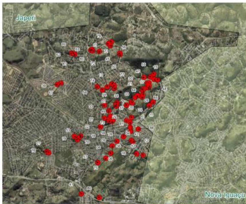
Figura 14 – Setores de risco iminente frente a deslizamentos (DRM-RJ, 2010).
