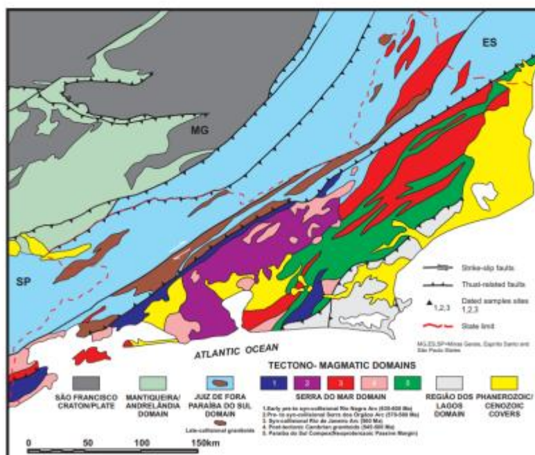
Figura 12 – Domínios tectono-magmáticos do Estado do Rio de Janeiro e áreas adjacentes (CPRM, 2018).
