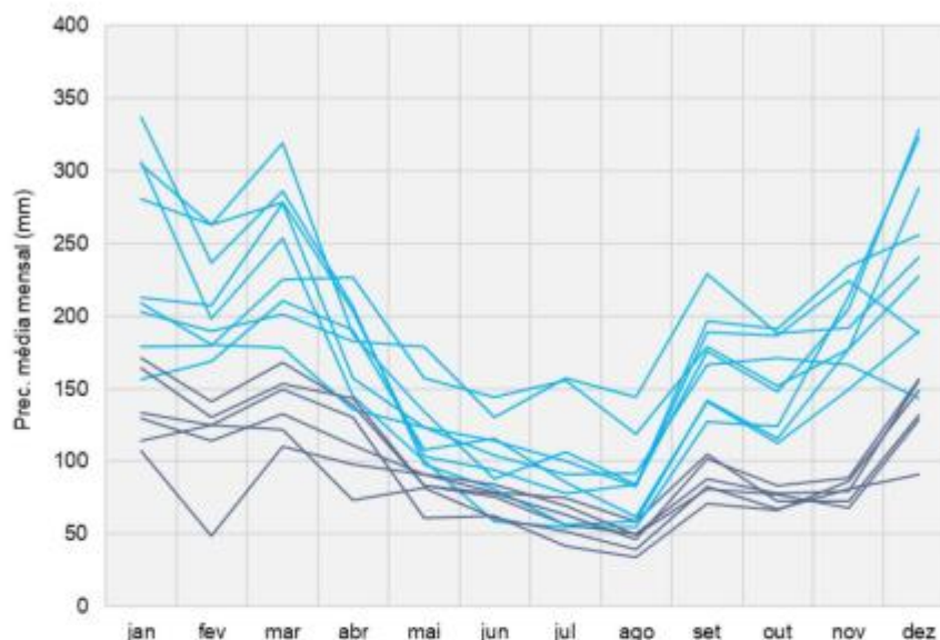
Figura 6 – Precipitação média mensal nos postos pluviométricos com dados disponíveis entre 1981 e 2000 (PERH Guandu, 2018).
