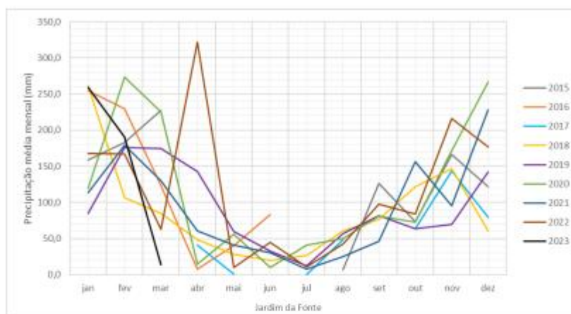
Figura 7 – Precipitação média mensal a partir de dados obtidos no CEMADEN.
