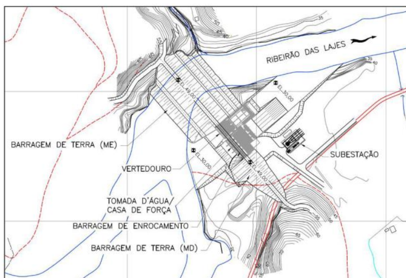
Figura 28 – Arranjo geral do barramento (Paracambi Energética, 2024).
